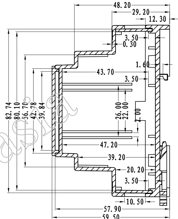
SEC A-A
