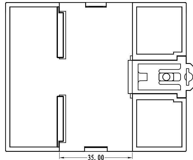
SEC A-A
