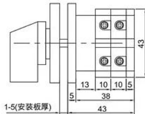
外形尺寸/Shape size
