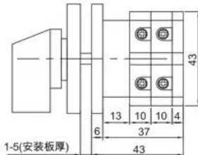
外形尺寸/Shape size
