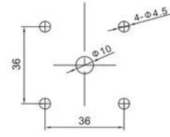
安装尺寸/Installation size
